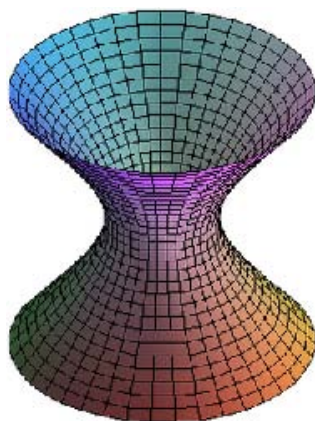
hiperboloide
