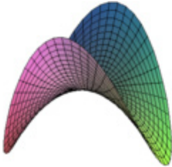
paraboloide hiperbòlic
